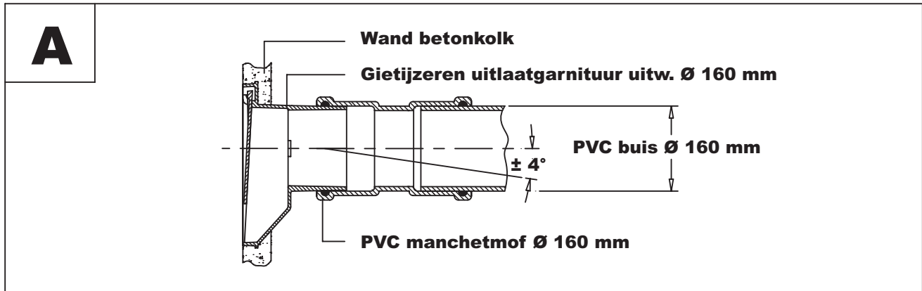
Aansluiting d.m.v. PVC manchetmof \varnothing 160 mm over spie-eind kolk
