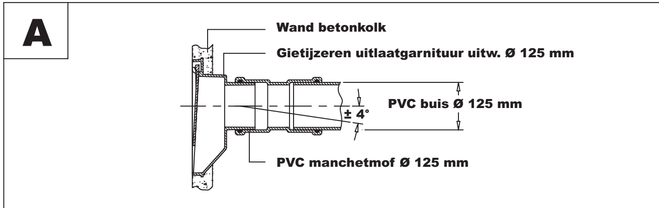
Aansluiting d.m.v. PVC manchetsmf \varnothing 125 mm over spie-eind kolk
