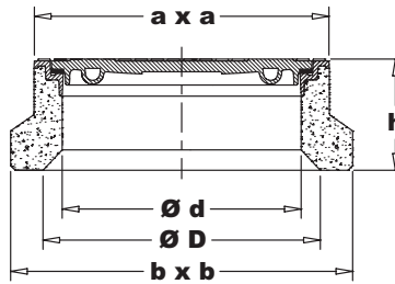
type N 352 NB-R Centerfix WADI 170 - 240 mm
